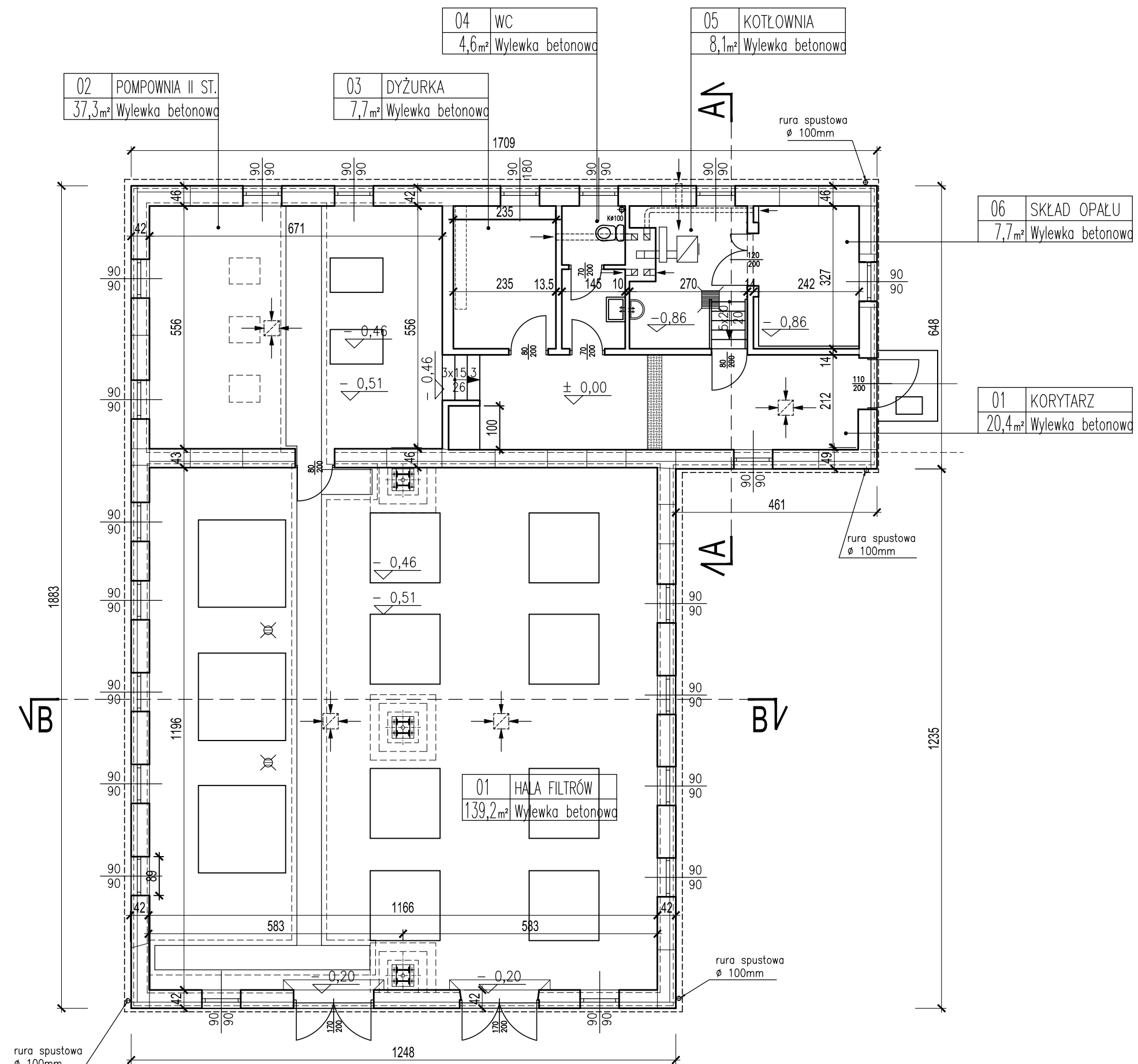
RZUT PRZYZIEMIA skala 1:100
