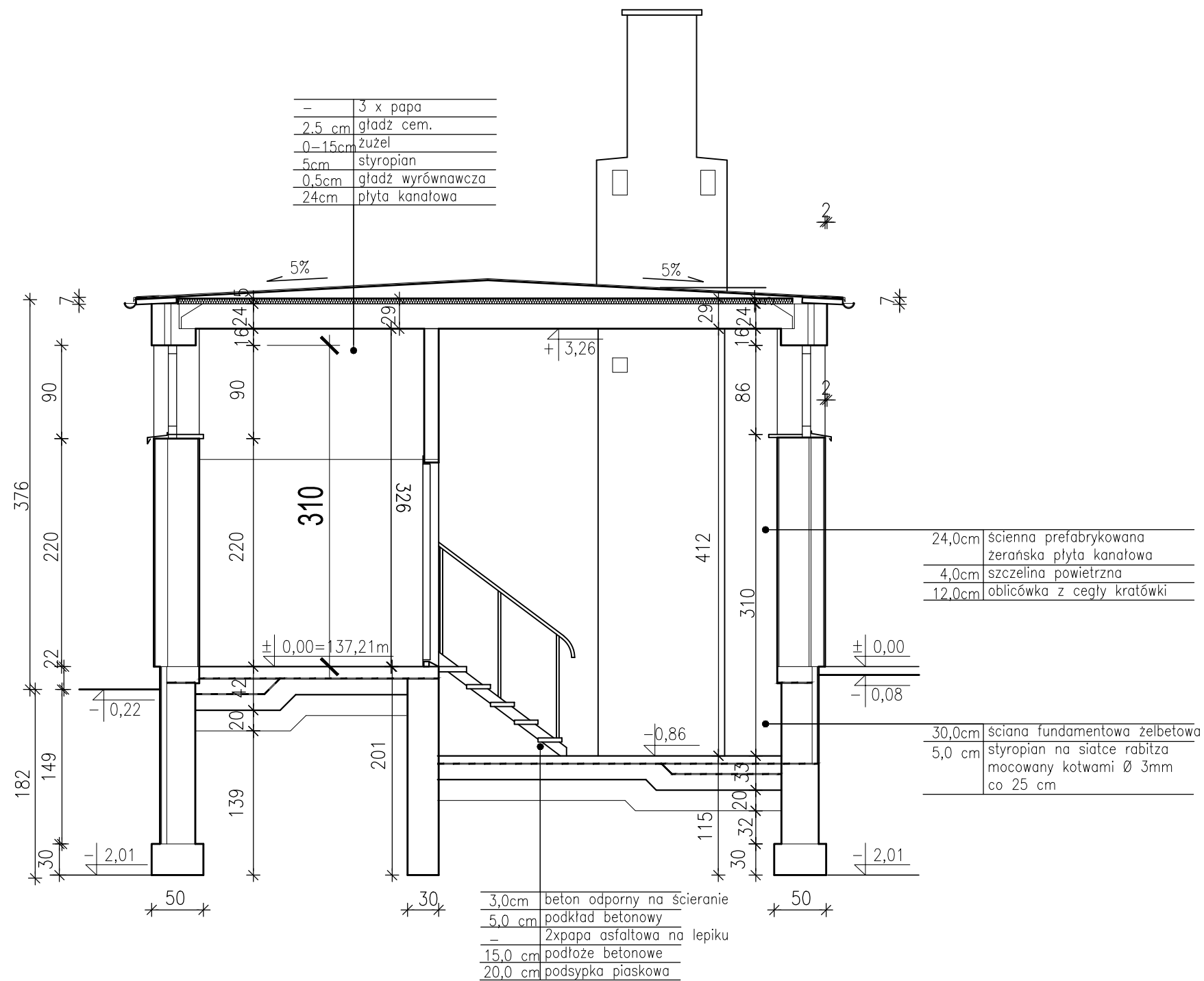
PRZEKRÓJ A-A skala 1:50
